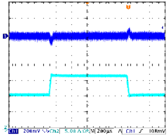
50%-75%-50%Io动态负载
