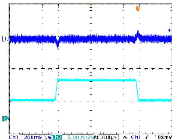
25%-50%-25%Io动态负载
