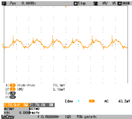
输出纹波
