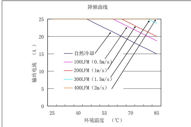
无散热器条件下的热交换曲线 (不同风速条件下输入电流与环境温度的关系, Vinom)
