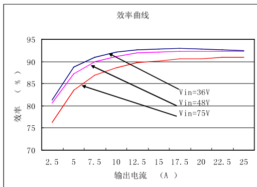
输出电流与效率关系曲线(Tc = +25°C)
