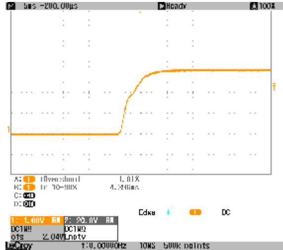
输出上升时间
