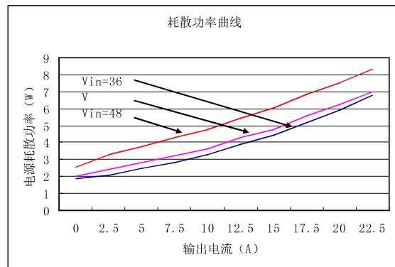
输出电流与损耗关系曲线
